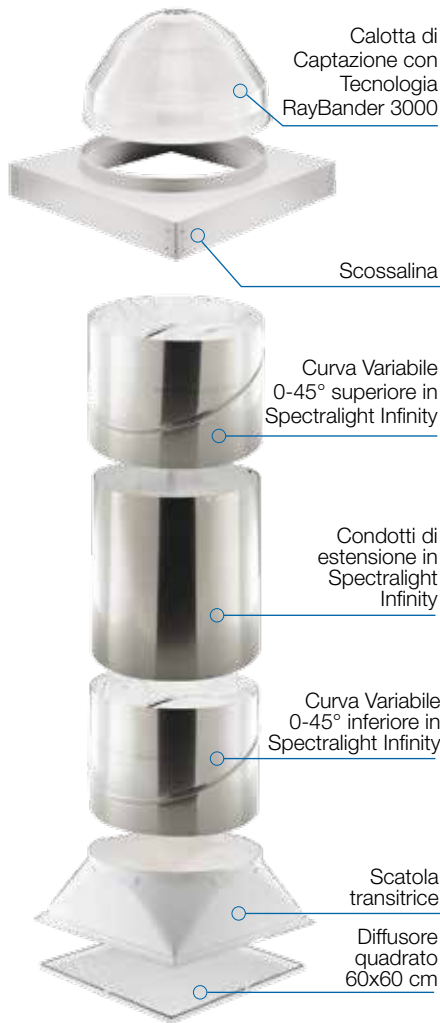
Solatube 750 DS
